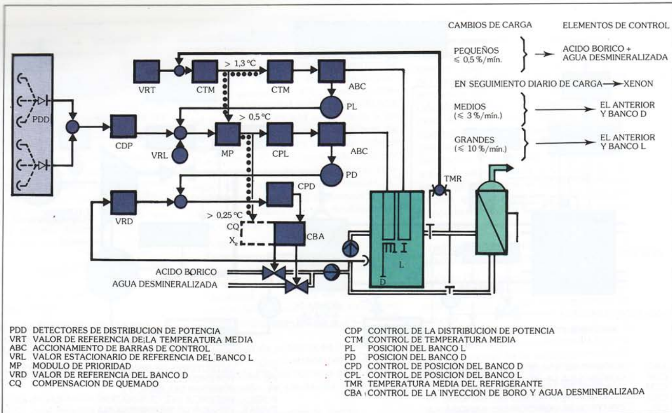
F XI Sistemas de control de potencia del reactor.
