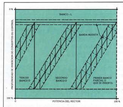
F XII Principio del control de barras. Esquema de inserción de barras de control.
