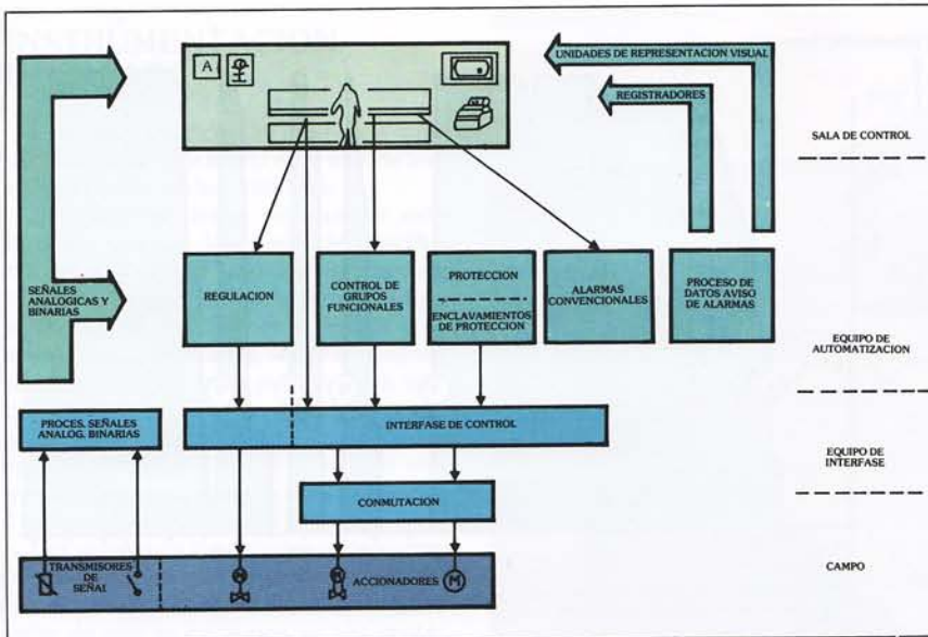
FIV Organización de la instrumentación y control de Servicio.
