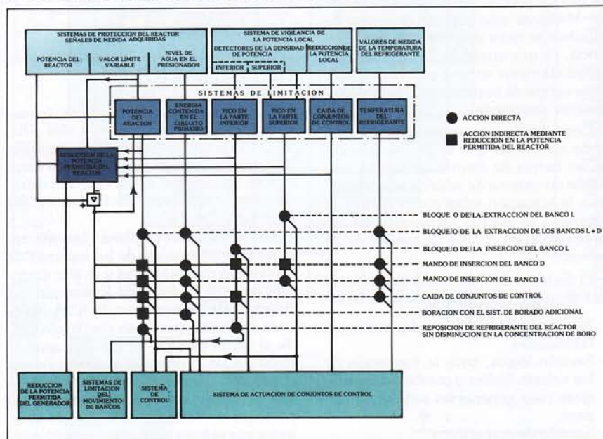
FIG IX Concepto de los Sistemas de Alimentación de la potencia del reactor.
