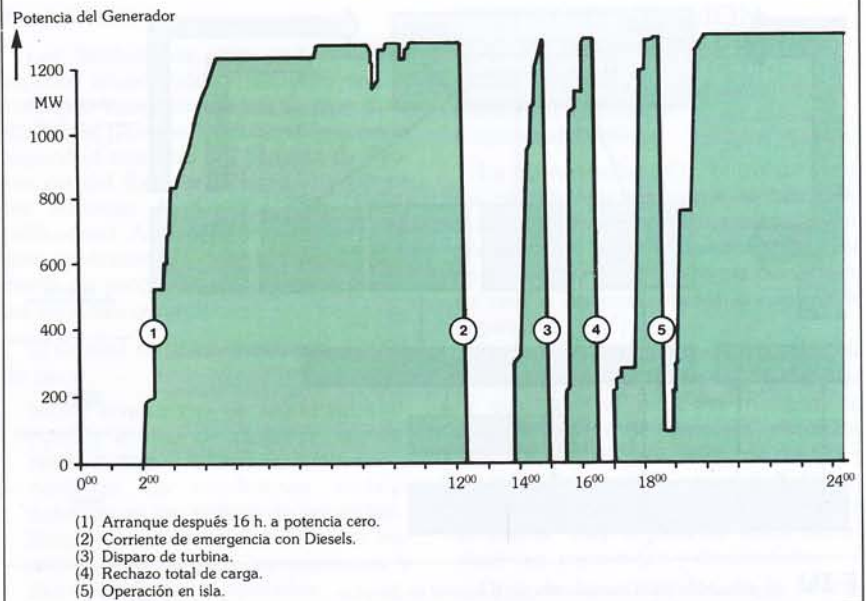
F VII Pruebas de arranques múltiples en una Central KWU.
