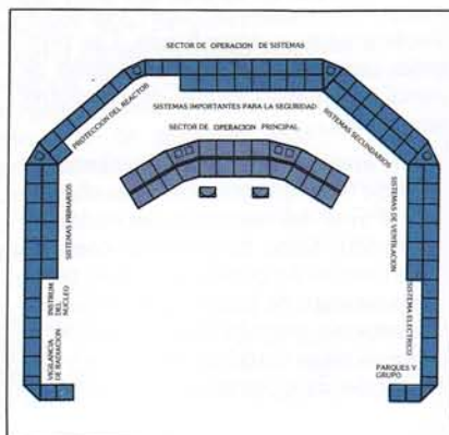
F XIII Sala de Control.
